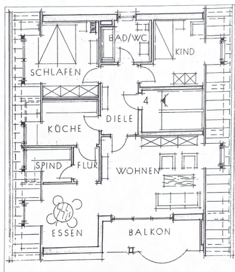
Grundriss
