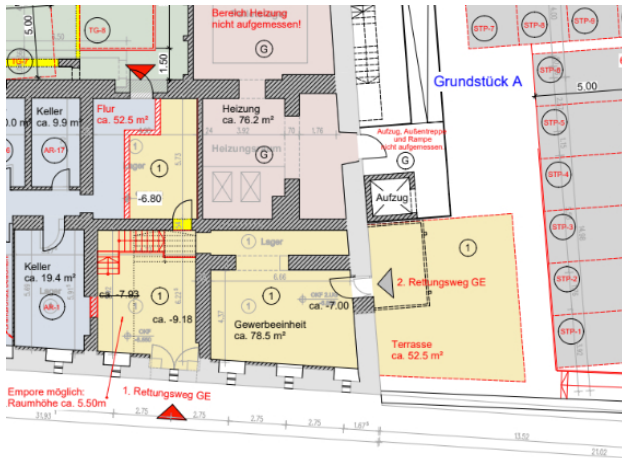
Grundriss_Gewerbe_Nr. 1_UG 2
